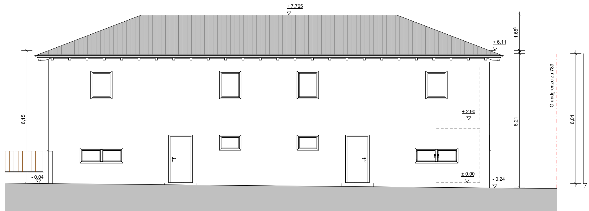
NORD-Ansicht
