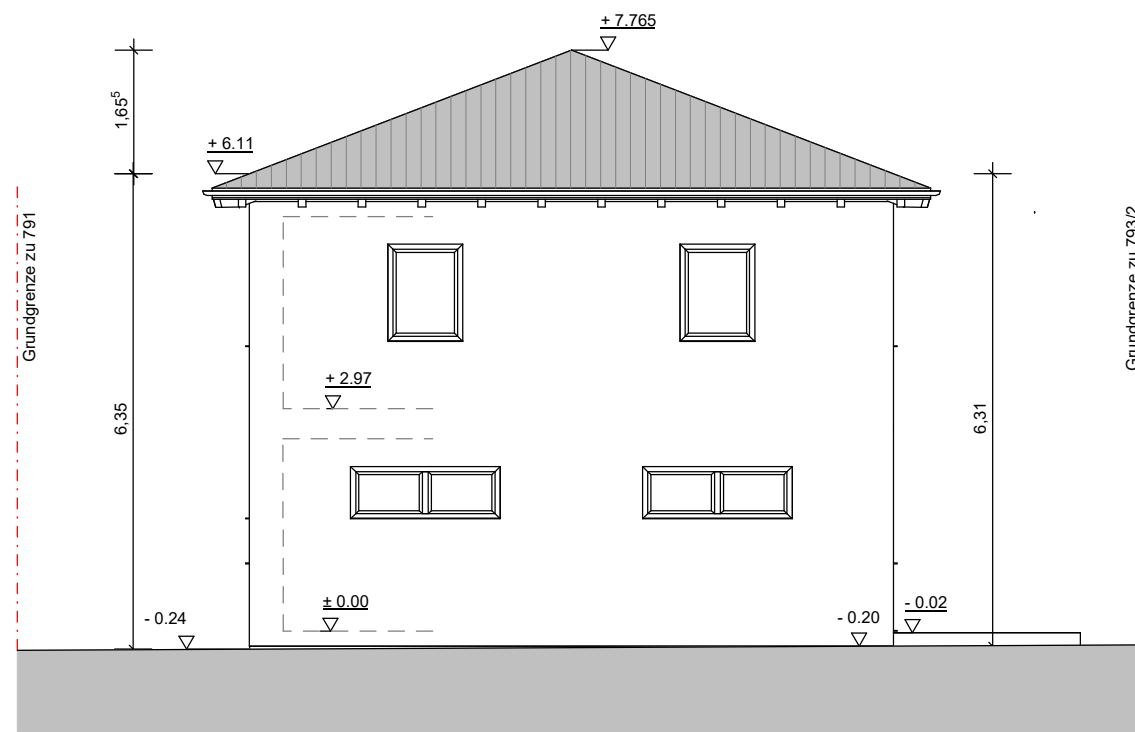
WEST-Ansicht
